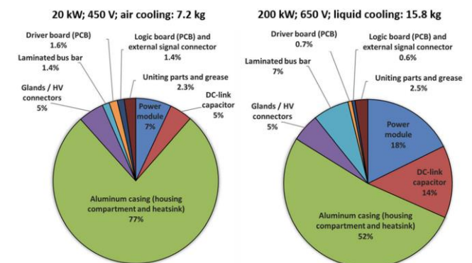
Fig. 4. Inventaire des composants présents dans deux onduleurs [5]
