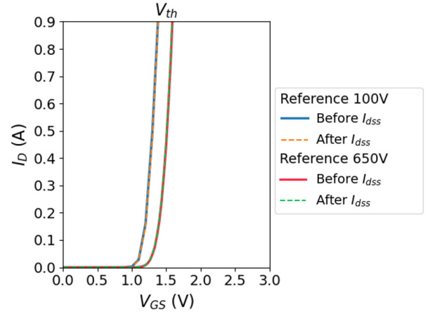
FIG. 4. Mesure V_{th} préconditionnée (à V_{GS,PC} = 7V ) avant et après une mesure I_{dss} pour un HEMT pGaN de 100 V et 650 V.
