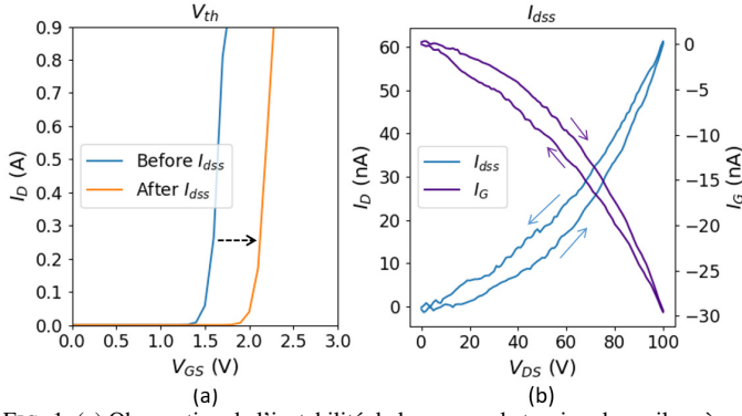
FIG. 1. (a) Observation de l'instabilité de la mesure de tension de seuil après une mesure I_{dss} avec V_{ds} jusqu'à 100V (b) Mesure de la fuite de courant à V_{GS} = 0V de le transistor pendant le I_{dss} qui provoque le décalage de V_{th} de (a) (balayages avant et arrière pointés par les flèches). Toutes les mesures ont été effectuées à une température ambiante de 20 °C. La vitesse de balayage est de 33 V/s.
