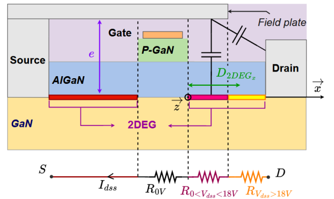
FIG. 11. Vue simplifiée du transistor et de l'emplacement du gaz d'électrons 2D pour un V_{DS} = V_{dss} donné. Le modèle équivalent du chemin de résistance est illustré ci-dessous. Les résistances rose ( R_{0V} ) et jaune ( R_{0V} < V_{dss} < 18 V) varient, R_{0V} est constante à l'état OFF.
