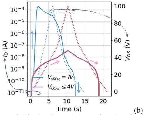
FIG. 9. Courant de fuite de drain pour plusieurs valeurs de tension de grille de préconditionnement appliquées auparavant, (a) en fonction de la tension de drain appliquée, (b) évolution dans le temps de la tension et du courant de drain. Comme le balayage est plus rapide que sur la Fig.7 (33V/s contre 3V/s), le pic de courant de fuite supplémentaire n'a pas le temps de s'évacuer uniquement sur la phase de balayage direct. Le courant supplémentaire du pic est évacué plus rapidement lors de la mesure avec un balayage plus rapide ( \approx 12 s contre 20 s sur la Fig.7), puisque la charge à évacuer est la même pour un même V_{GS,PC} , le courant maximal atteint est plus élevé à des vitesses de balayage plus rapides.
