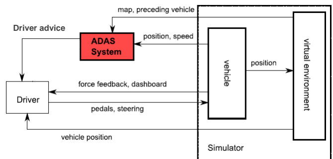
Fig.11 Schéma global de la configuration expérimentale
